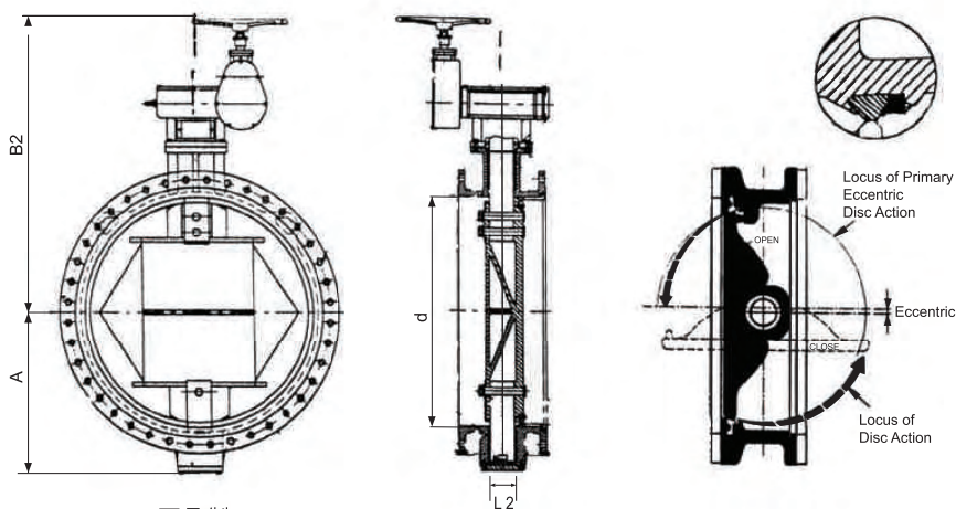
可承製48"
