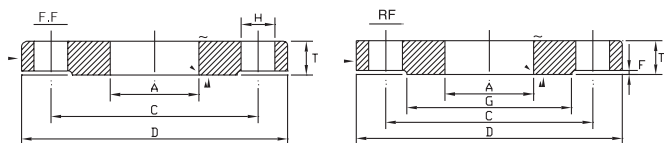
ANSI 300型 FLANGES
