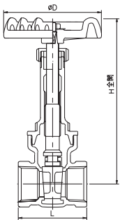
單位/mm
