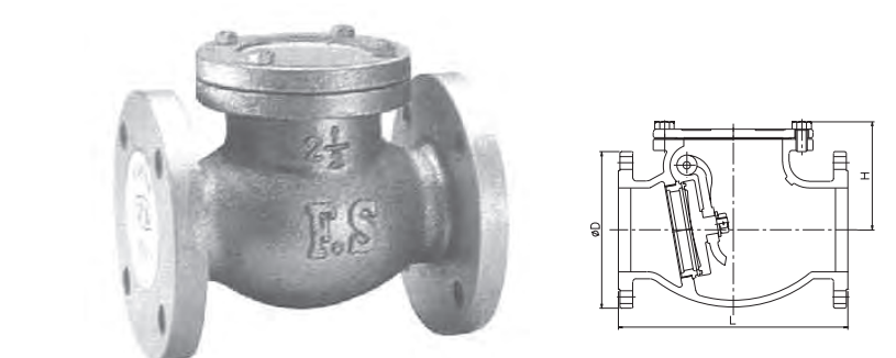
註: JIS-20K產品, 編號 FS-012PA3 單位/mm
