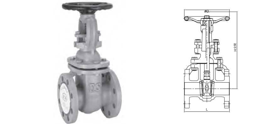
註: JIS-20K產品, 編號 FS-011PA3 單位/mm
