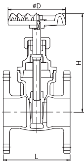
單位/mm
