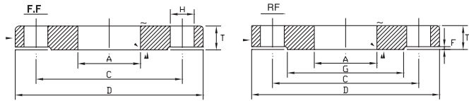
ANSI 150型 FLANGES
