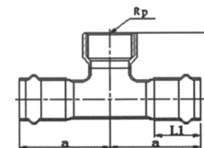
代號:YMO 平管橋 Q
