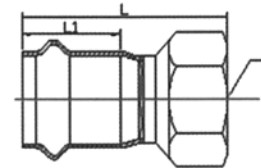
代號:YMSS 水栓接頭WS
