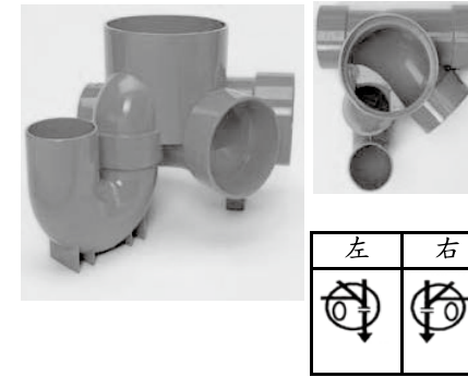
單接糞管及存水彎側通匯流井(45YS-UT)
