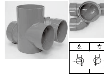
單接糞管側通匯流井(HYS)
