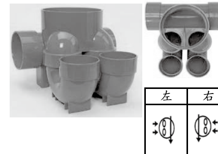
雙接存水彎匯流井(UTW)
