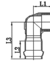
代號:YMAEM 外牙彎頭90AE-M
