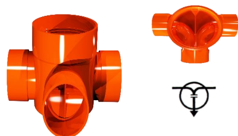
兩側合流匯流井(WLS)
