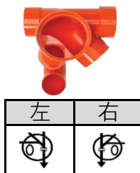
單接糞管及存水彎側通匯流井(45YS-UT)
